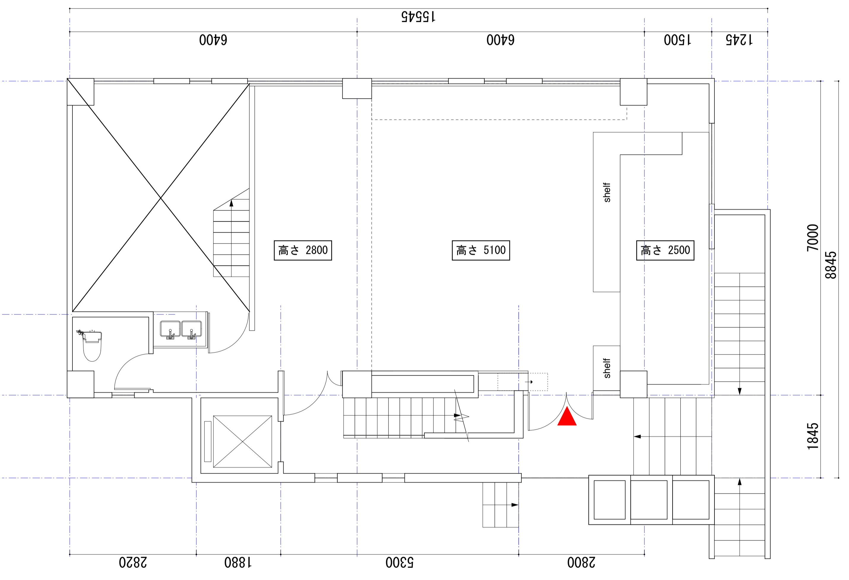
図面 (平面)
